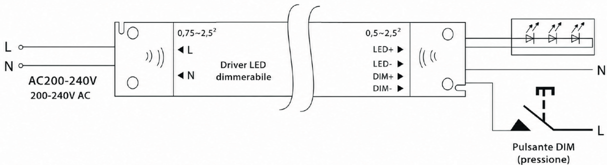
Schema di collegamento con comando PUSH
