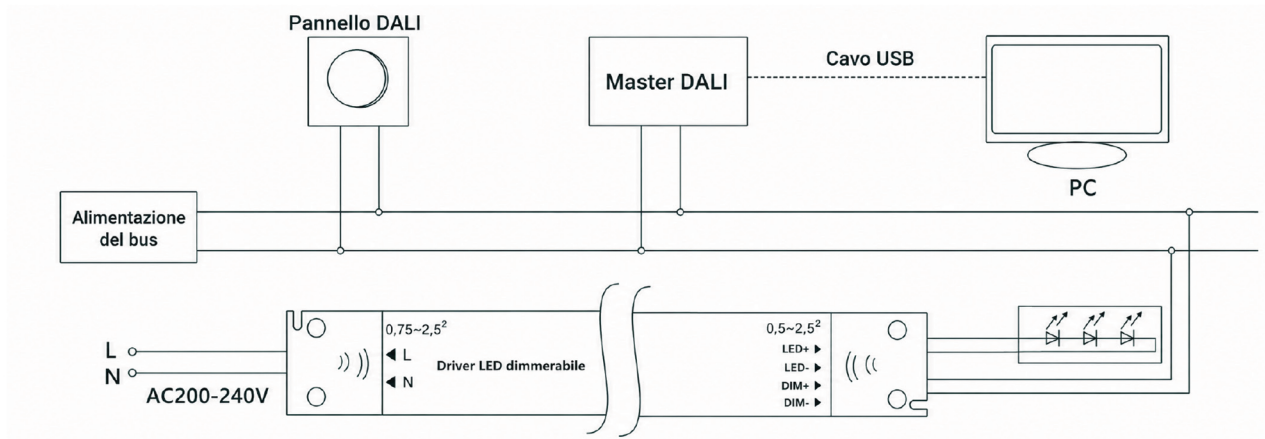
Schema di collegamento per la regolazione DALI
